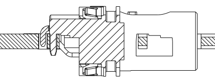
SCHNITT D-D SECTION D-D
