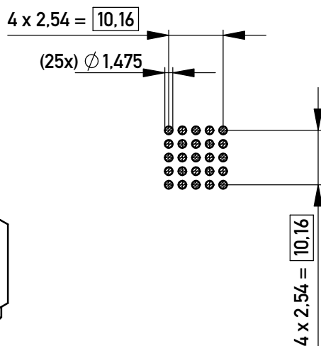
Layout - Vorschlag PCB - Layout proposal M 1:1 scale 1:1
