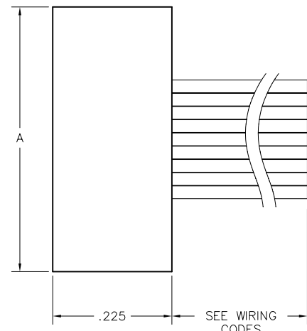
RECEPTACLE
