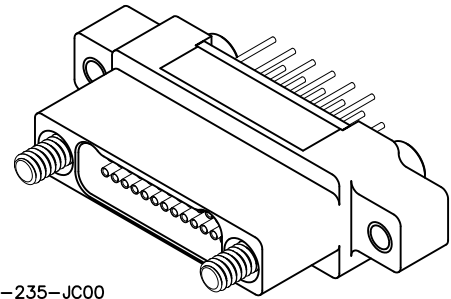
NK-2N2-025-235-JC00 RECEPTACLE
