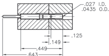
RECEPTACLE
