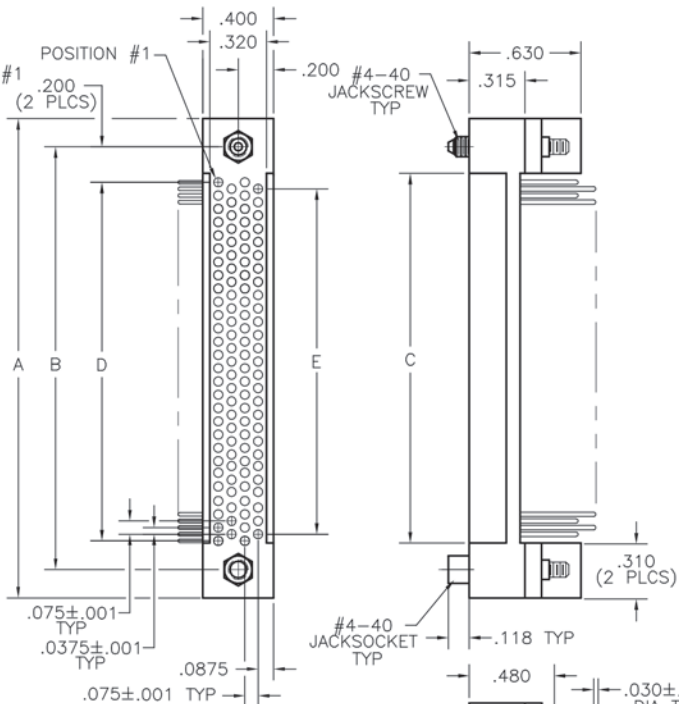
RECEPTACLE
