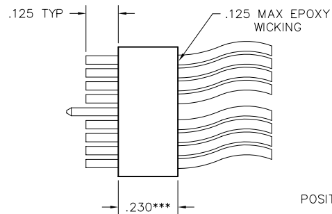
RECEPTACLE
