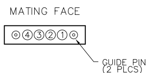
RECEPTACLE MA-141-004-261-A67WA
