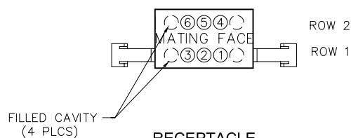
RECEPTACLE MA-241-006-261-A51WA
