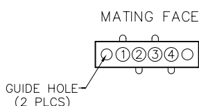
PLUG MA-1H1-004-145-A6800
