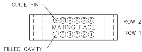
RECEPTACLE MA-221-010-261-A63WA
