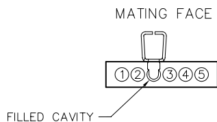
PLUG MA-131-005-161-A03WA
