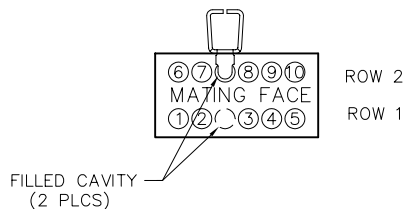
PLUG MA-231-010-161-ABCWA
