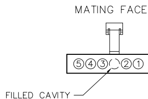
RECEPTACLE MA-141-005-261-A03WA
