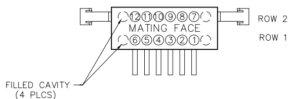
RECEPTACLE MA-2C1-012-435-A5300
