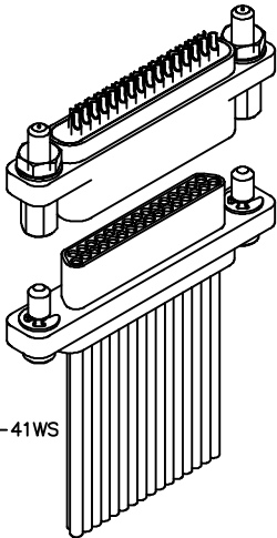
MQHT-222-031-2A3-2200 (METAL)
