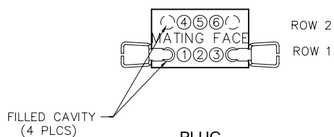
PLUG MA-231-006-161-A50WA
