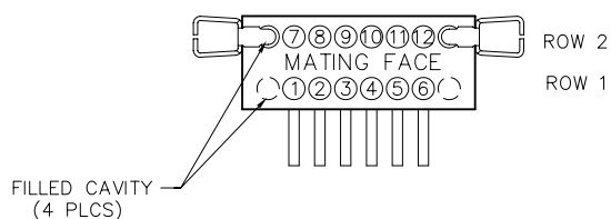
PLUG MA-2B1-012-325-A5200
