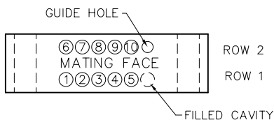
PLUG MA-211-010-161-A66WA
