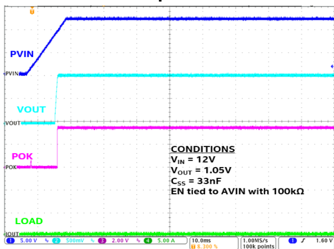
VIN Startup at No Load
