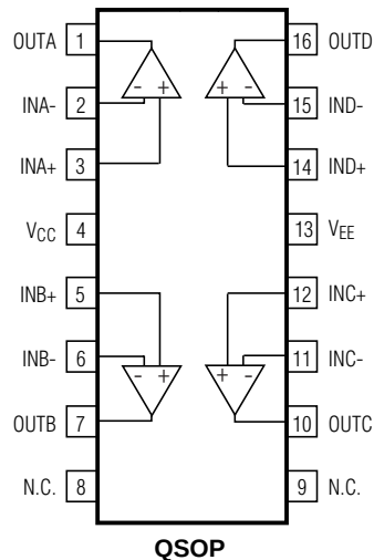
MAXIM MAX4284
