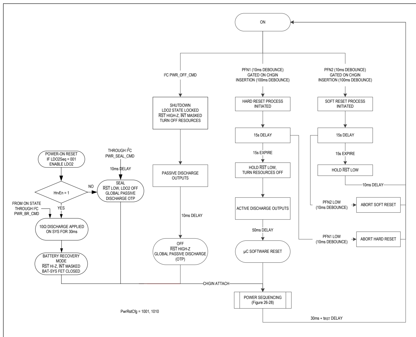
Figure 21. PwrRstCfg 1001, 1010
