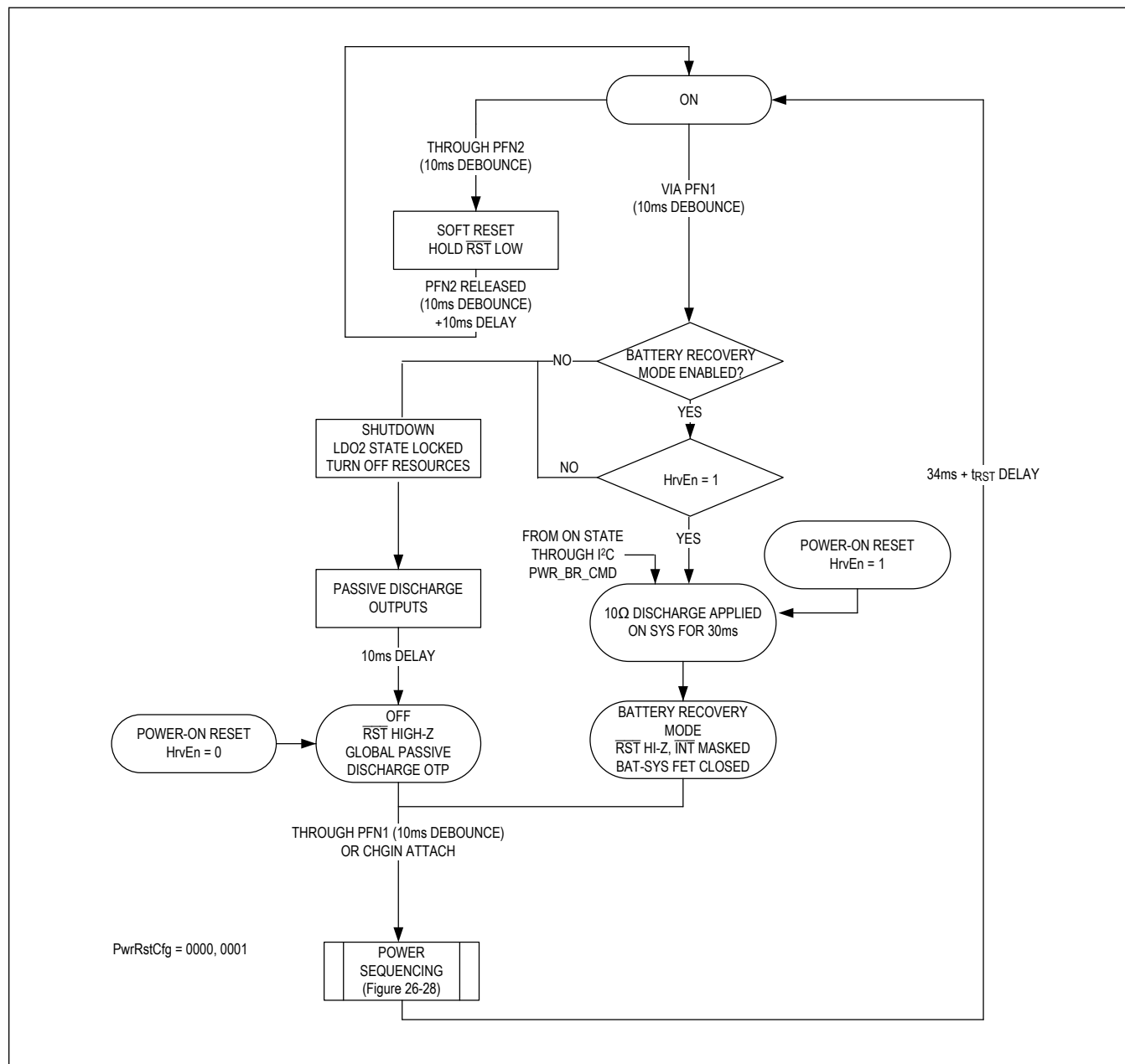
Figure 15. PwrRstCfg 0000, 0001
