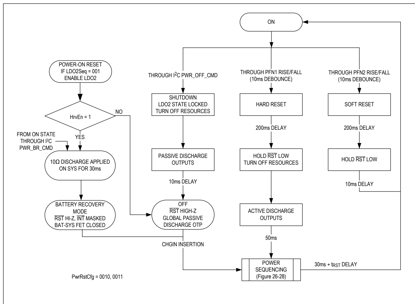
Figure 16. PwrRstCfg 0010, 0011
