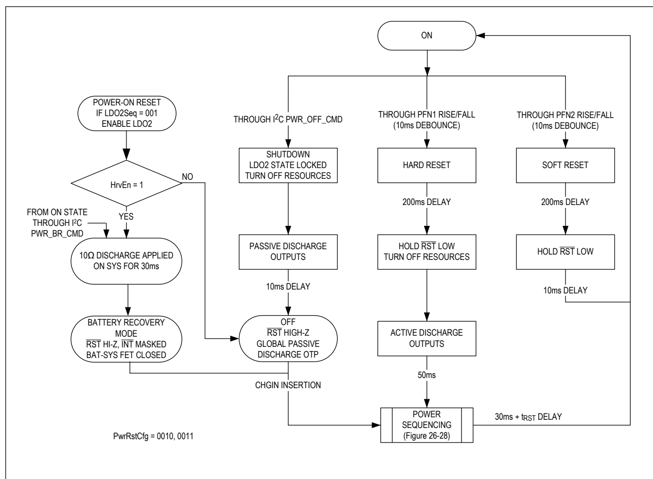
Figure 16. PwrRstCfg 0010, 0011
