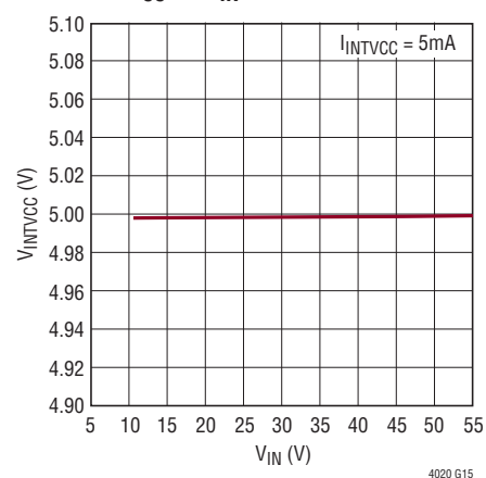
V_{INTVCC} vs V_{IN}
