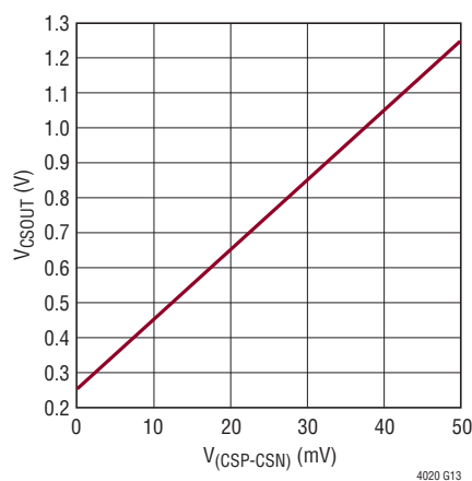
CSOUT vs CSP-CSN
