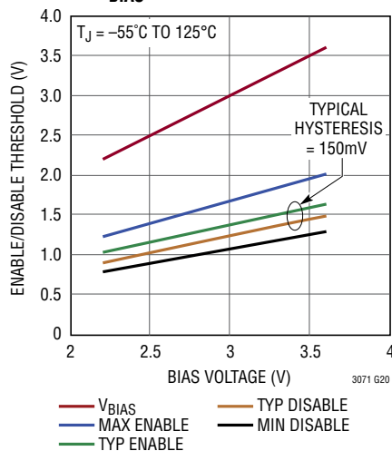
EN Pin Threshold and Hysteresis vs V_{BIAS}
