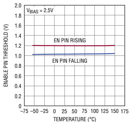
EN Pin Thresholds
