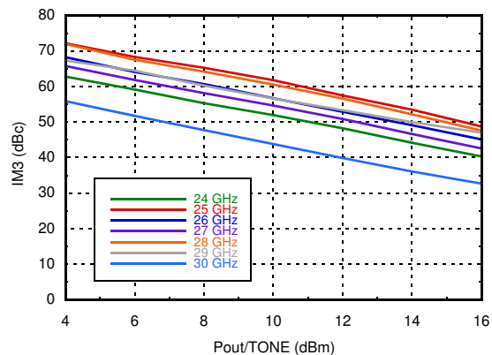
Output IM3
