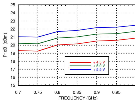
P1dB vs. Vdd
