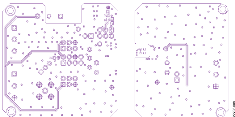
Figure 9. EVAL-ADM2565EEBZ/EVAL-ADM2865EEBZ, Layer 2
