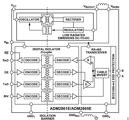
Figure 2. ADM2861E/ADM2865E
