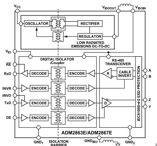
Figure 1. ADM2863E/ADM2867E
