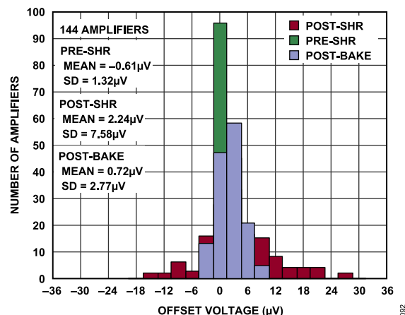
Figure 92. V_{OS} Shift due to Solder Heat
