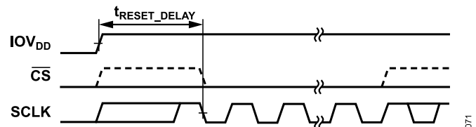
Figure 70. POR Timing Diagram
