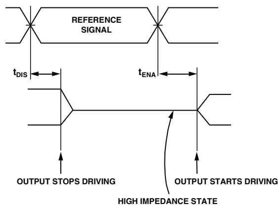
Figure 28. Output Enable/Disable
