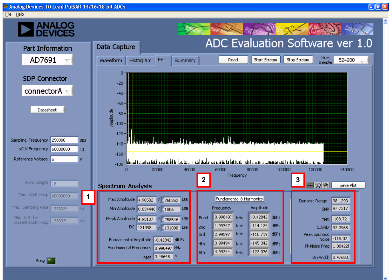
Figure 24. FFT Tab
