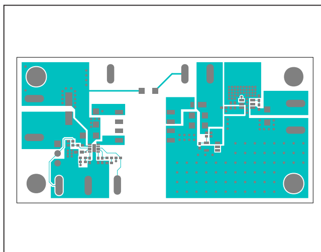
MAX17681 EV Kit—Top Layer
