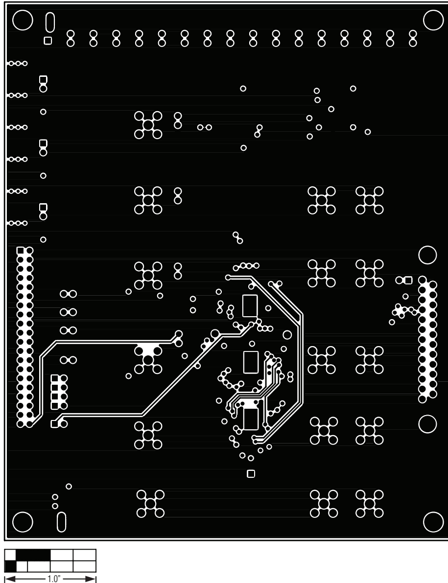
Figure 5. MAX13171E/MAX13173E/MAX13175E EV Kit PCB Layout—Inner Layer 3
