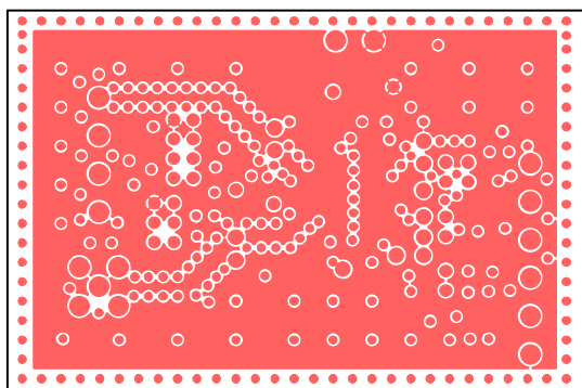
Figure 7. EVAL-ADM3067EEBZ, Layer 3
