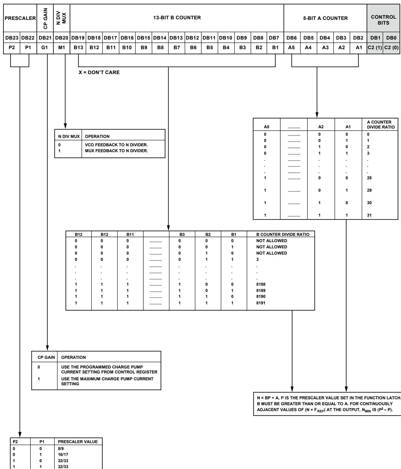
Figure 25. LO Latch
