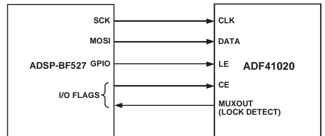
Figure 19. ADSP-BF527-to-ADF41020 Interface
