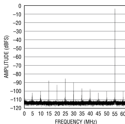
LTM9012, 125Msps, 70MHz FFT
