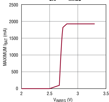
Maximum I_{\text{BAT}} vs V_{\text{INREG}}
