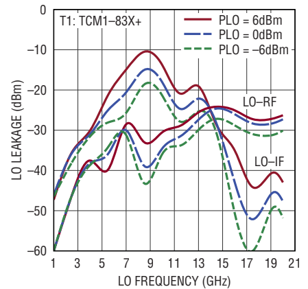
LO Leakage
