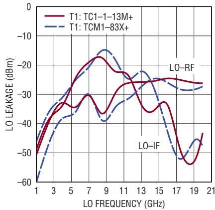
LO Leakage
