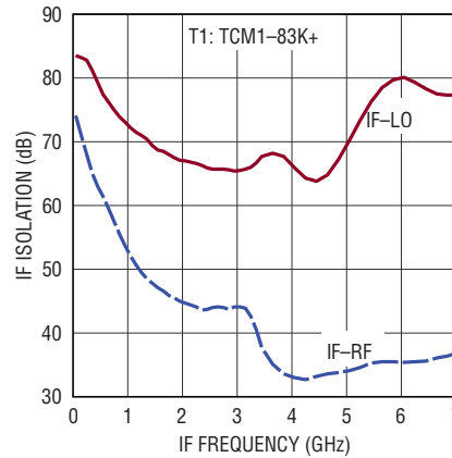
IF Isolation
