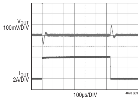
2.5V Load Transient
