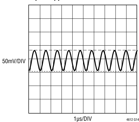
Input Ripple
