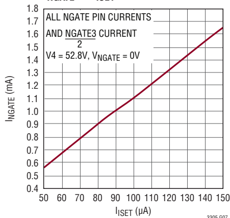
I NGATE vs I ISET
