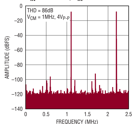
32k Point FFT, IMD, f_{\text{SMPL}} = 5\text{Msps} , A_{\text{IN}}^+ = 1.2\text{MHz} , A_{\text{IN}}^- = 2.2\text{MHz}
