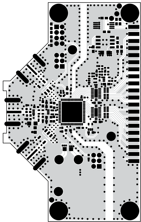
Top Side
