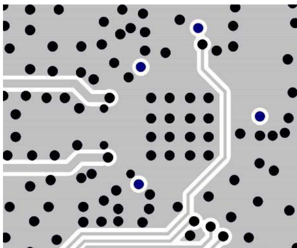
Bottom Side
