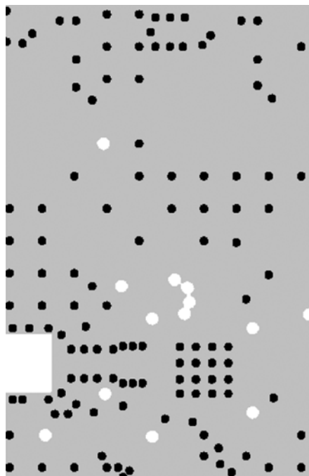
Inner Layer 2
