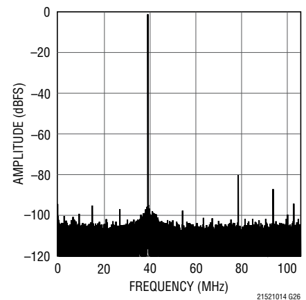
LTC2151-14: 32K Point FFT, f_{IN} = 171\text{MHz} , -1\text{dBFS} , 210Mps
