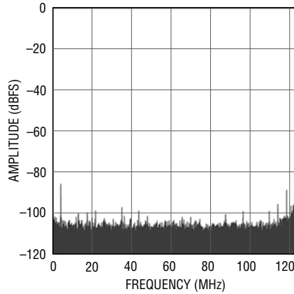
LTC2152-14: 32K Point FFT, f_{IN} = 122\text{MHz} , -1\text{dBFS} , 250\text{Mps}
