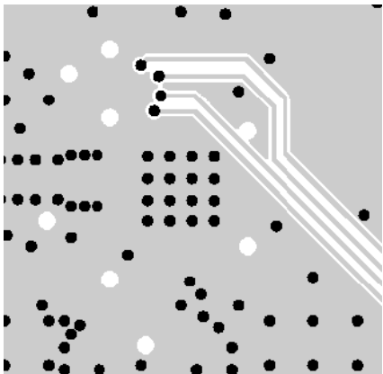
Inner Layer 3
