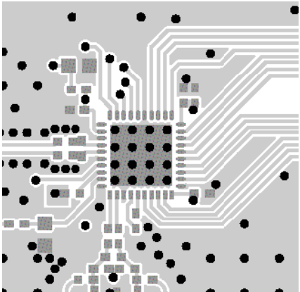
Inner Layer 1
