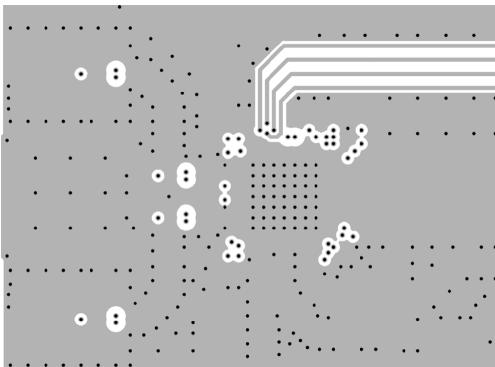
Inner Layer 4
