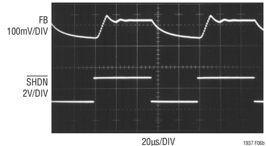
(6b) 10kHz
