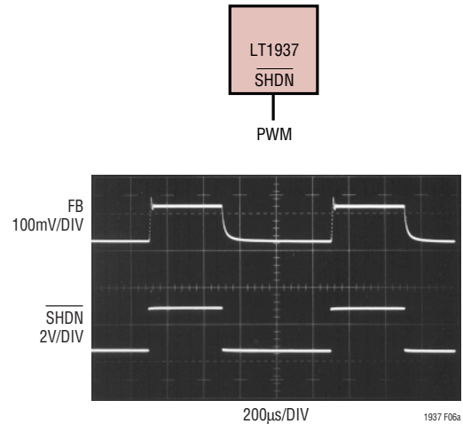
(6a) 1kHz
