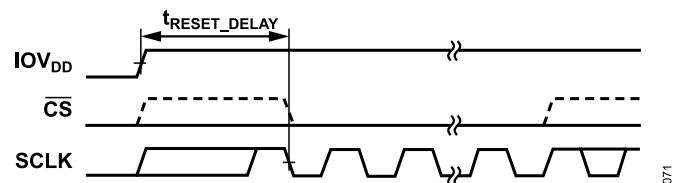
Figure 68. POR Timing Diagram
