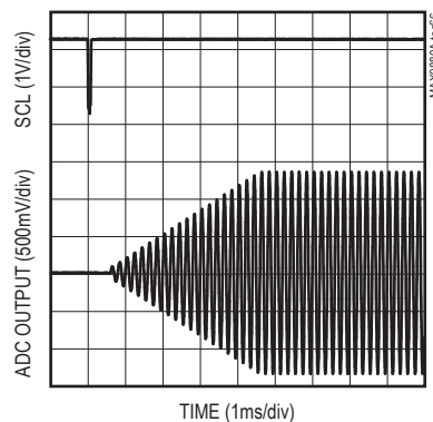
SOFT-START ADC
