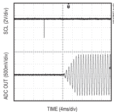
ADC SOFT-START
