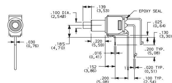
TP12SH9AVBE SPDT
