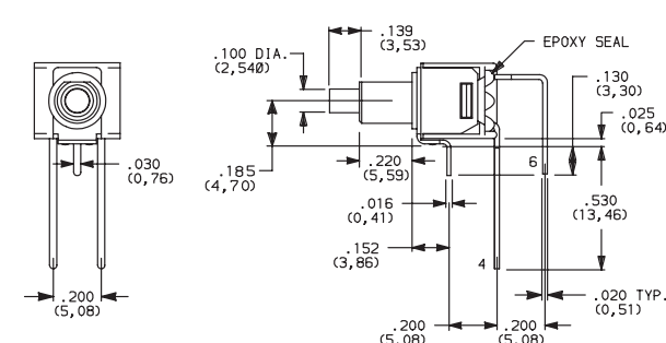
TP21SH9AVBE DPST
