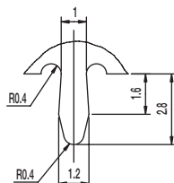
K DETAIL 2:1
