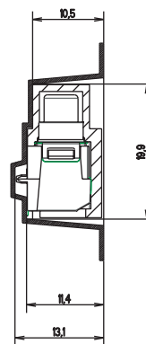
COUPE A-A
