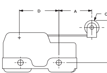
FIG. 1 Lever Roller
