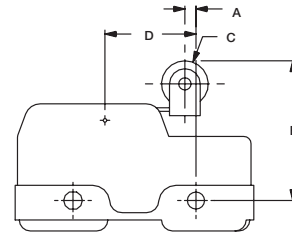
FIG. 2 Lever Roller
