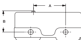
FIG. 5 Pin Plunger
