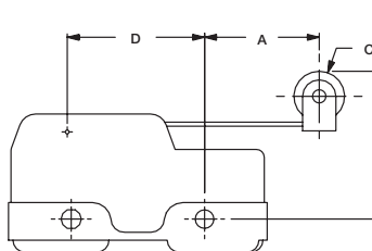
FIG. 1 Lever Roller
