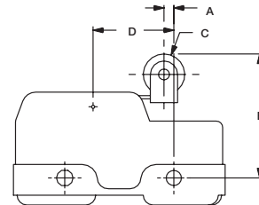
FIG. 2 Lever Roller
