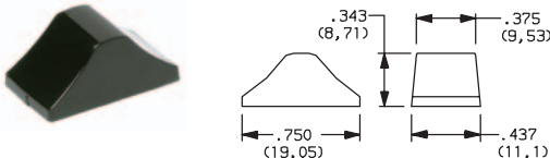
Cap, 03 actuator
