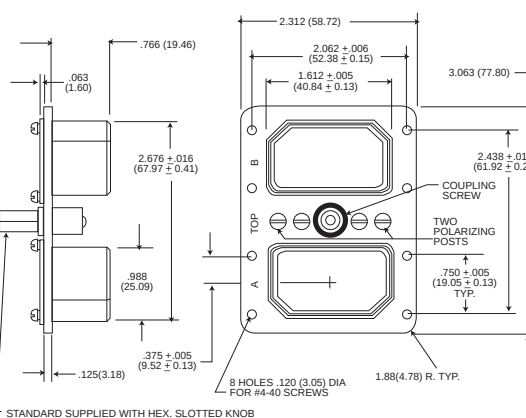
DPX2-33M (Male)
