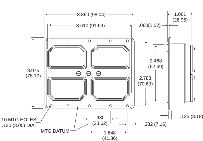
DPX4-34
