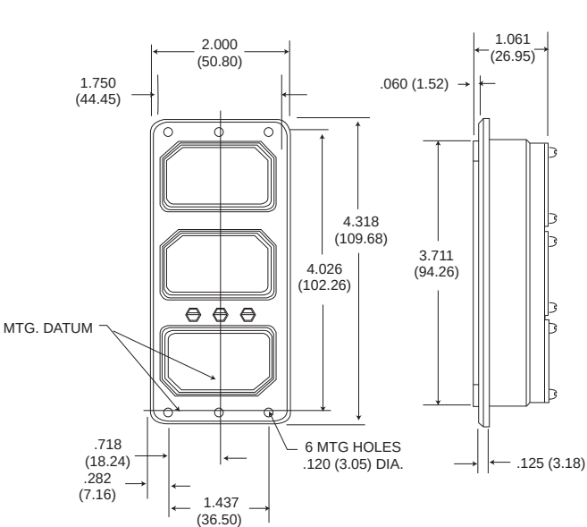
DPX3-34
